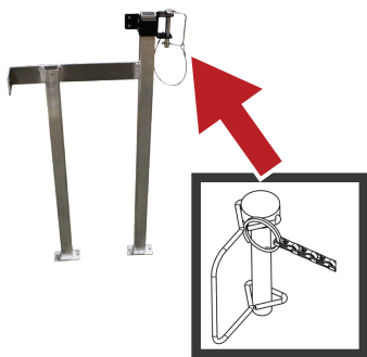
FWD CART BRACE Left Part#: 5018-006 Right Part#: 5018-007
